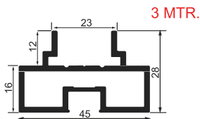
Door Profile Top / Bottom
