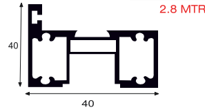
Door Rebate
