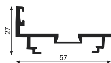
Door Rebate
