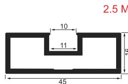
Door Frame Profile
