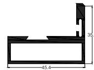
Door Rebate
