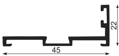
Door Rebate
