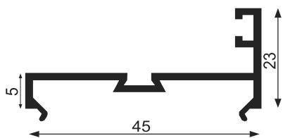
Door Rebate
