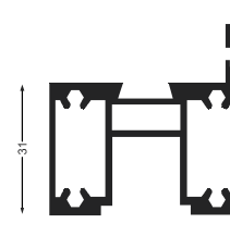
Door Outer Frame
