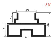
Door Profile Top / Bottom
